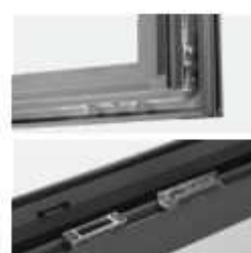
Renvoi d'angle avec galets champignon et gâches de sécurité anti-arrachement
