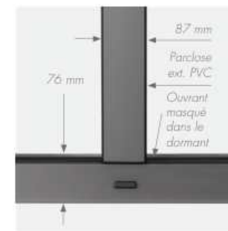
Ouvrant look carré réduit et masqué dans le dormant
